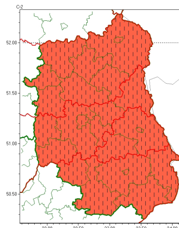
Upał 2026-08-01 06:05
