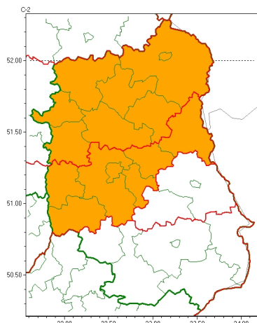
Burze 2026-08-01 06:05
